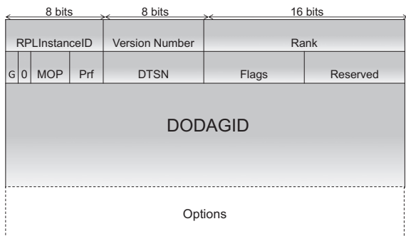
Fig. 3. The DIO message format.
